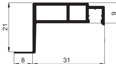
10 24 07.21 Spannrahmenprofil
