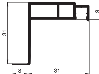
10 24 07.31 Spannrahmenprofil
