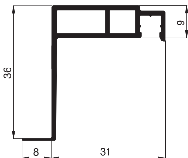
10 24 07.36 Spannrahmenprofil
